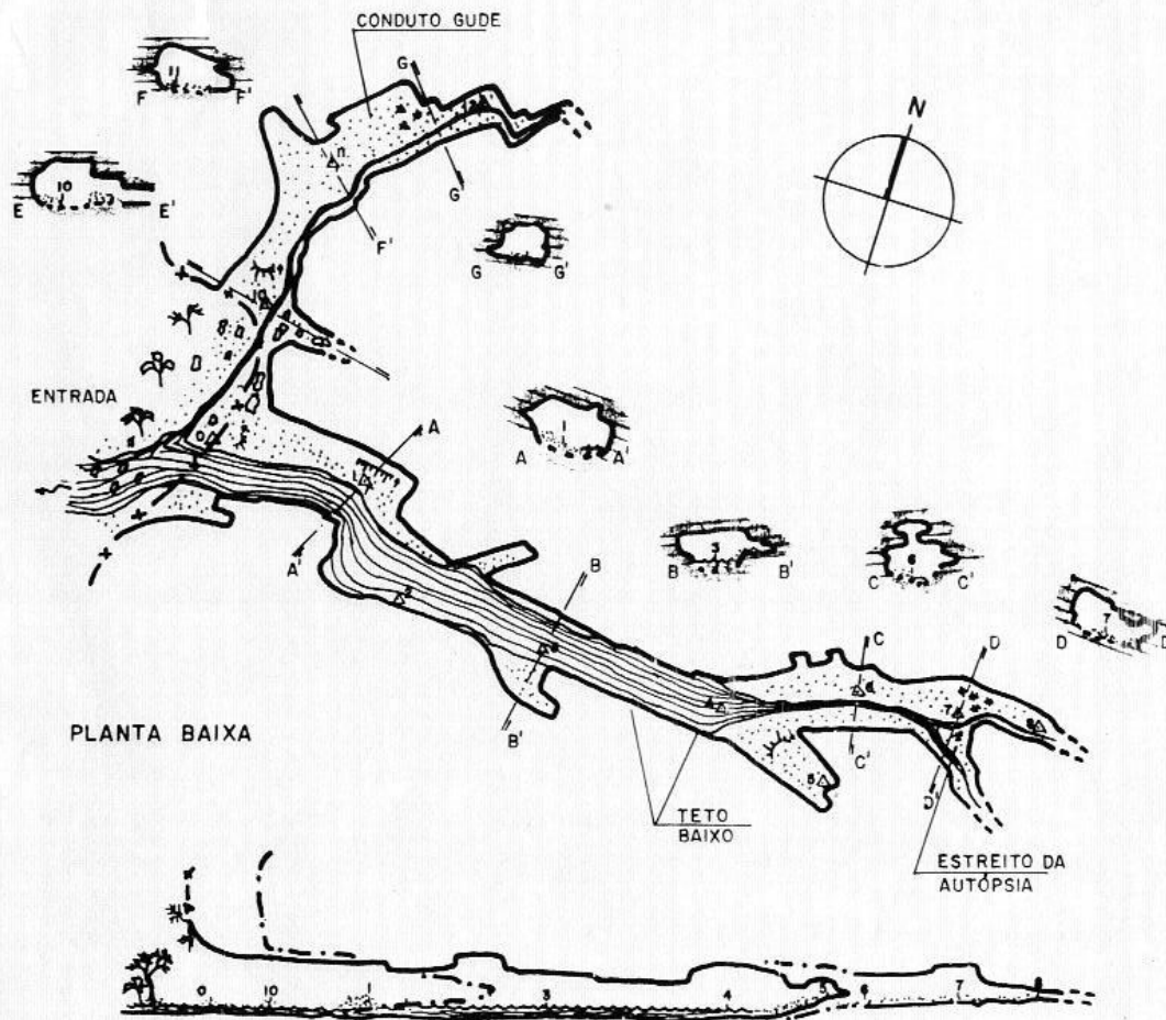
PERFIL LONGITUDINAL (W - E)
